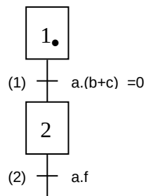
Transition validée non franchissable
