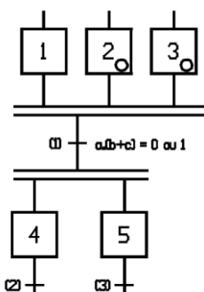
Transition (1) non validée
