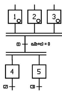
Transition (1) validée non franchissable
